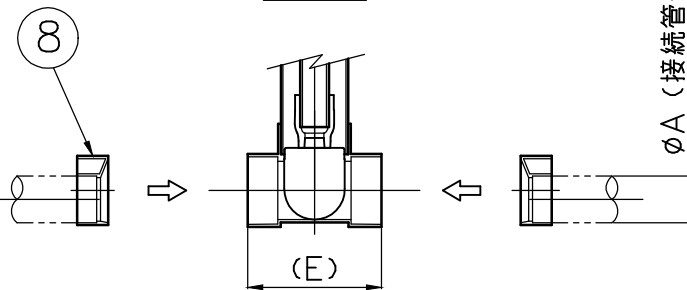
D2C-50・65の場合
