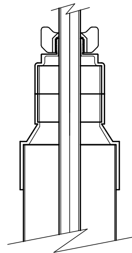
D2C-125・150の場合
