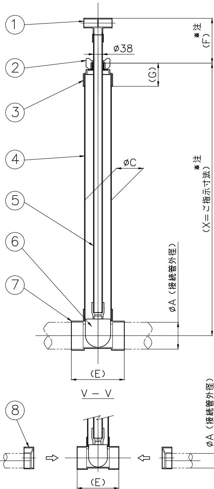
D2C-50・65の場合
