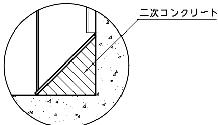
P部詳細
