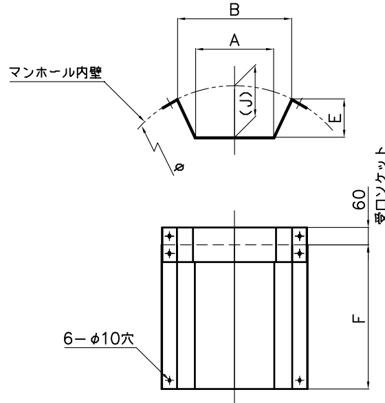
飛散防止板 TB (2)
