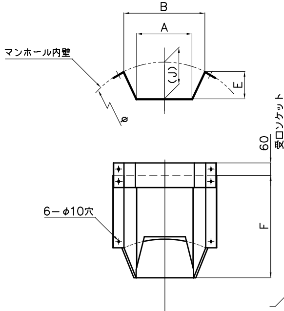
飛散防止板受台 TC (3)
