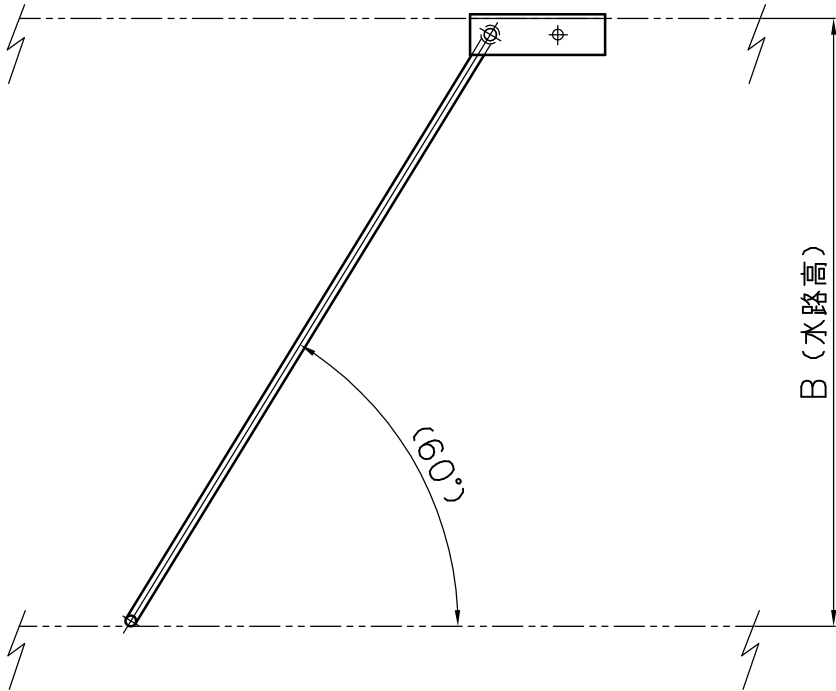
据付参考図
