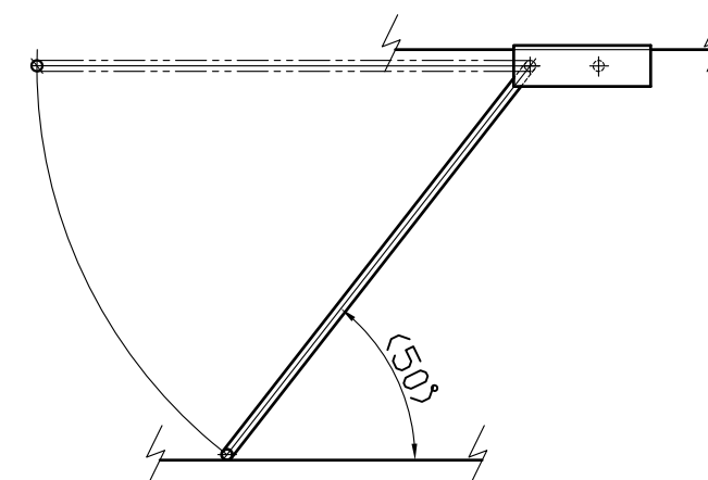
取 付 図
