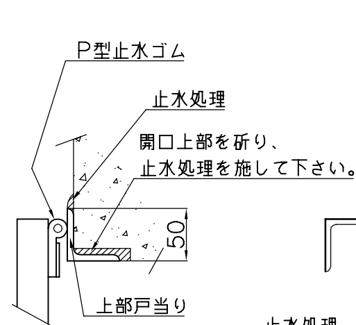
上部戸当り止水部詳細図 有効幅700~1000
