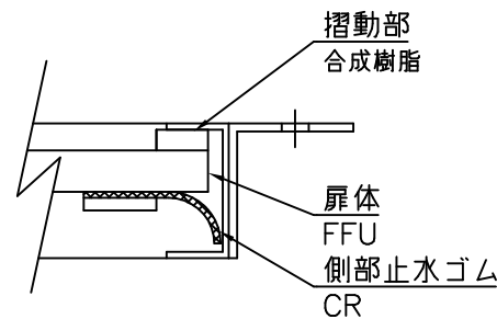
側部水密部 詳細図
