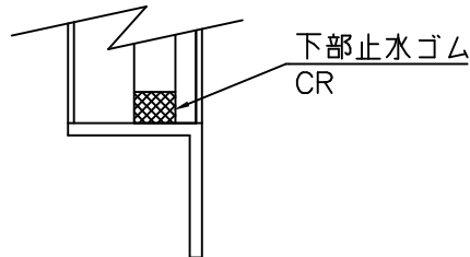
下部水密部 詳細図
